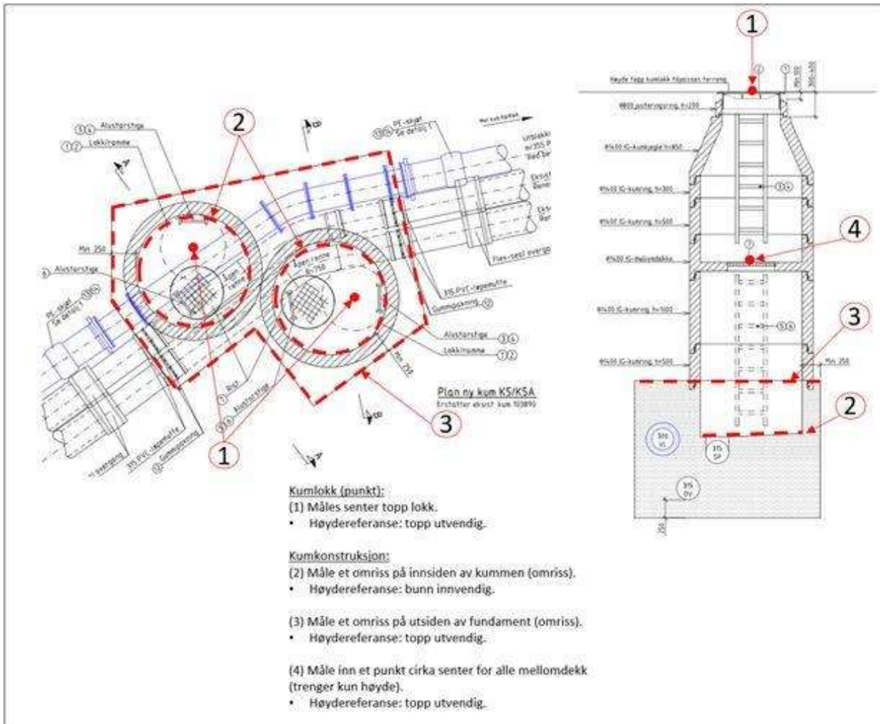
Figur 11: Innmåling av rundkummer.
