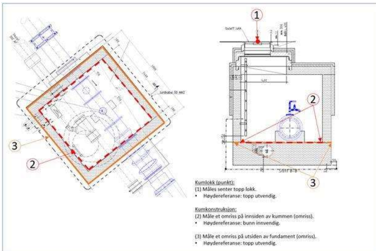
Figur 12. Innmåling av firkantkummer.
